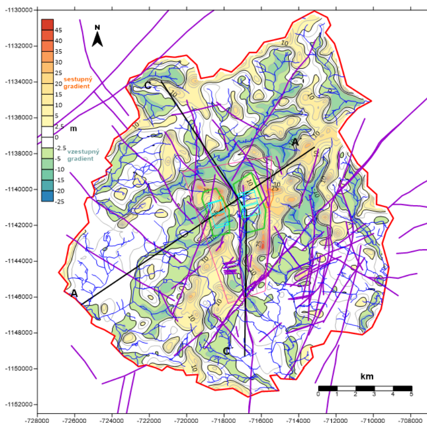
Obr. 10: Rozdíl modelové hladiny v připovrchové vrstvě a hladiny v úrovni HÚ (8 m n.m.), linie řezů A-A a C-C
