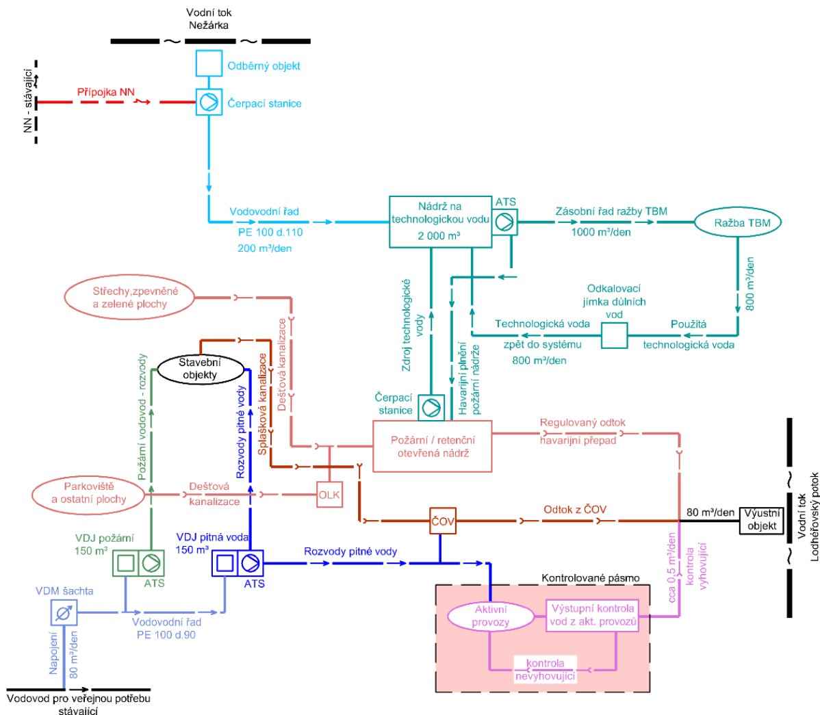
Obr. 57: Schéma vodního hospodářství HÚ
