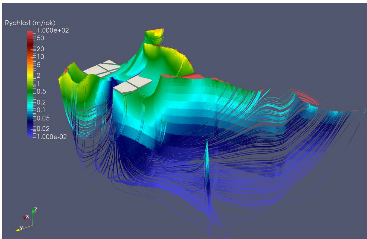
Obr. 17: Trajektorie particle trackingu z oblasti homogenních bloků s barevným rozlišením podle okamžité vypočtené rychlosti
