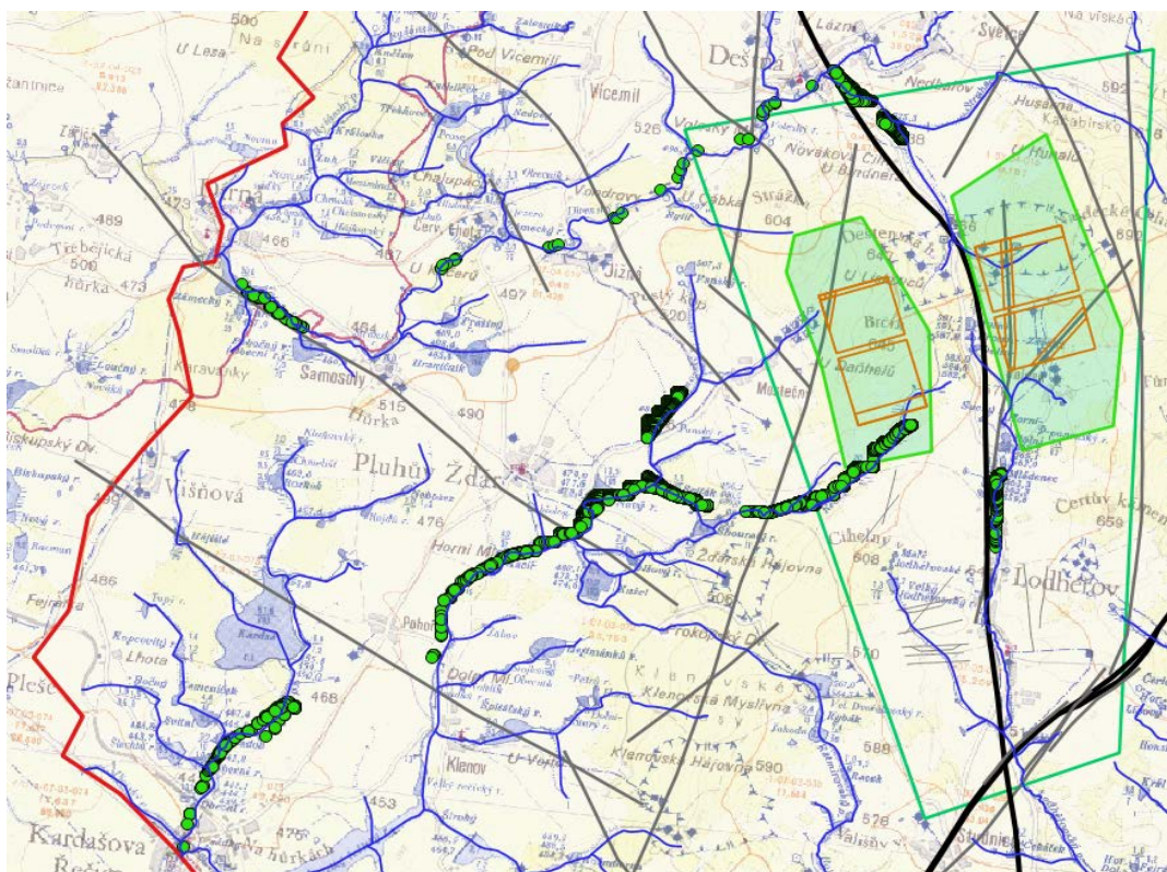
Obr. 12: Vypočtená místa drenáže pro podzemní vodu z projektovaného HÚ
