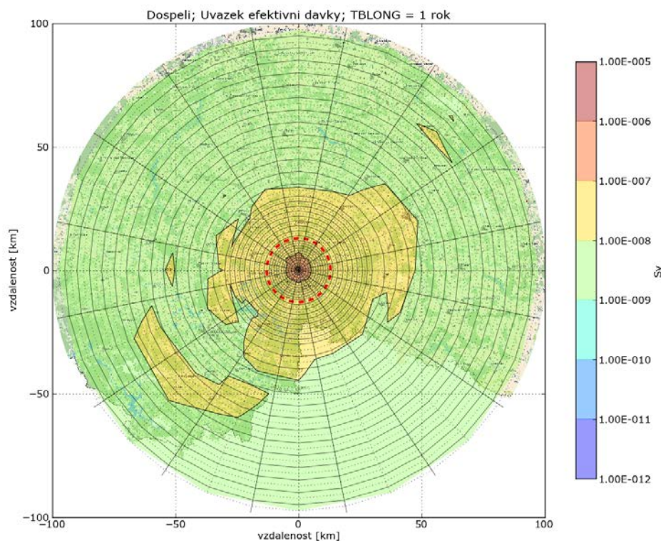
Obr. 30: Vypočet celkové expozice (efektivní dávka z externího ozáření a úvazek efektivní dávky z vnitřního ozáření) pro 16 směrů větrné růžice a referenčního dospělého jedince. (reprezentativní jedinec)
