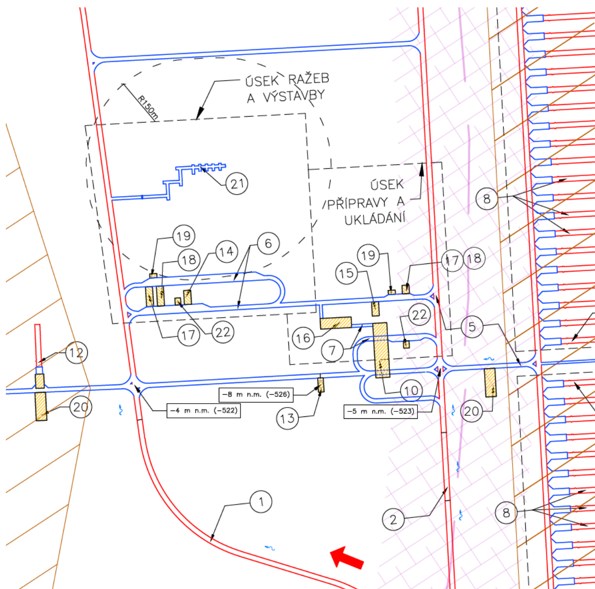
Obr. 62: Schéma technického zázemí (D1)
