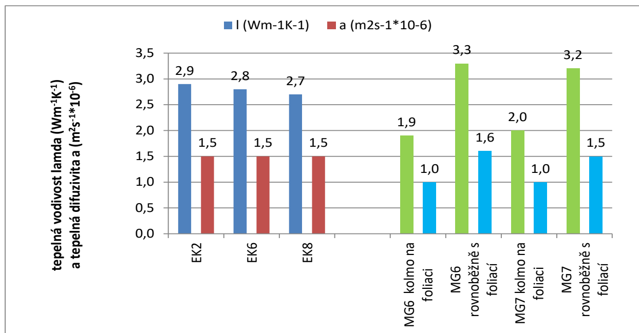
Obr. 23: Tepelná vodivost a tepelná difuzivita u granitů typu Klenov (EK) a migmatitů (MG) – lokalita Čihadlo
