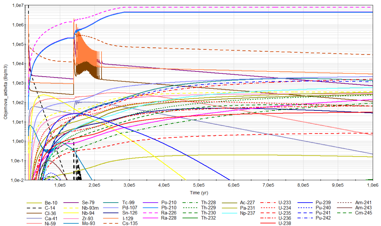
Obr. 40: Objemová aktivita radionuklidů uvolněných z blízkého pole (Bq/m 3 )
