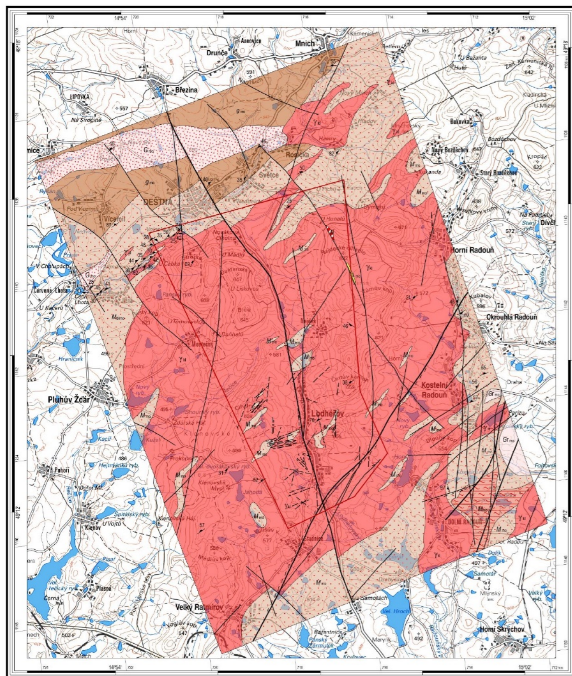
ČESKÁ GEOLOGICKÁ SLUŽBA ÚČELOVÁ GEOLOGICKÁ MAPA KANDIDÁTSKÉ LOKALITY ČIHADLO 1 : 50 000
