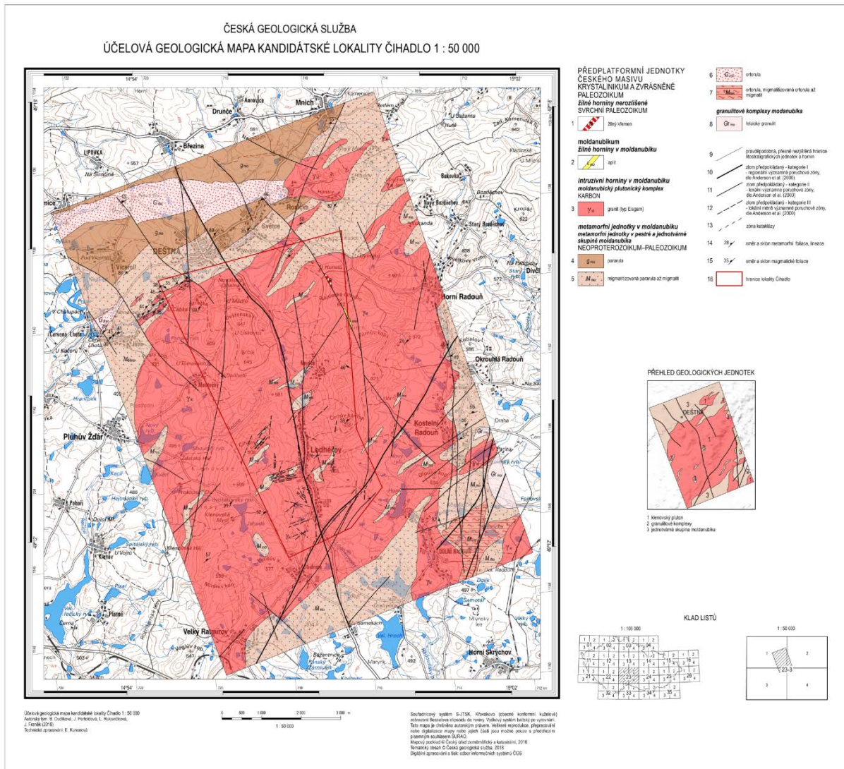
Obr. 5: Náhled na Účelovou geologickou mapu lokality Čihadlo
