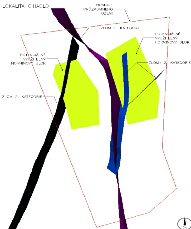
Obr. 3: Geologické schéma umístění využitelných horninových bloků v lokalitě Čihadlo
