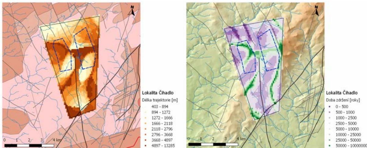
Obr. 18: Délky trajektorií a doby zdržení pro částice z prostoru vymezeného průzkumného území z úrovně 50 m n.m.
