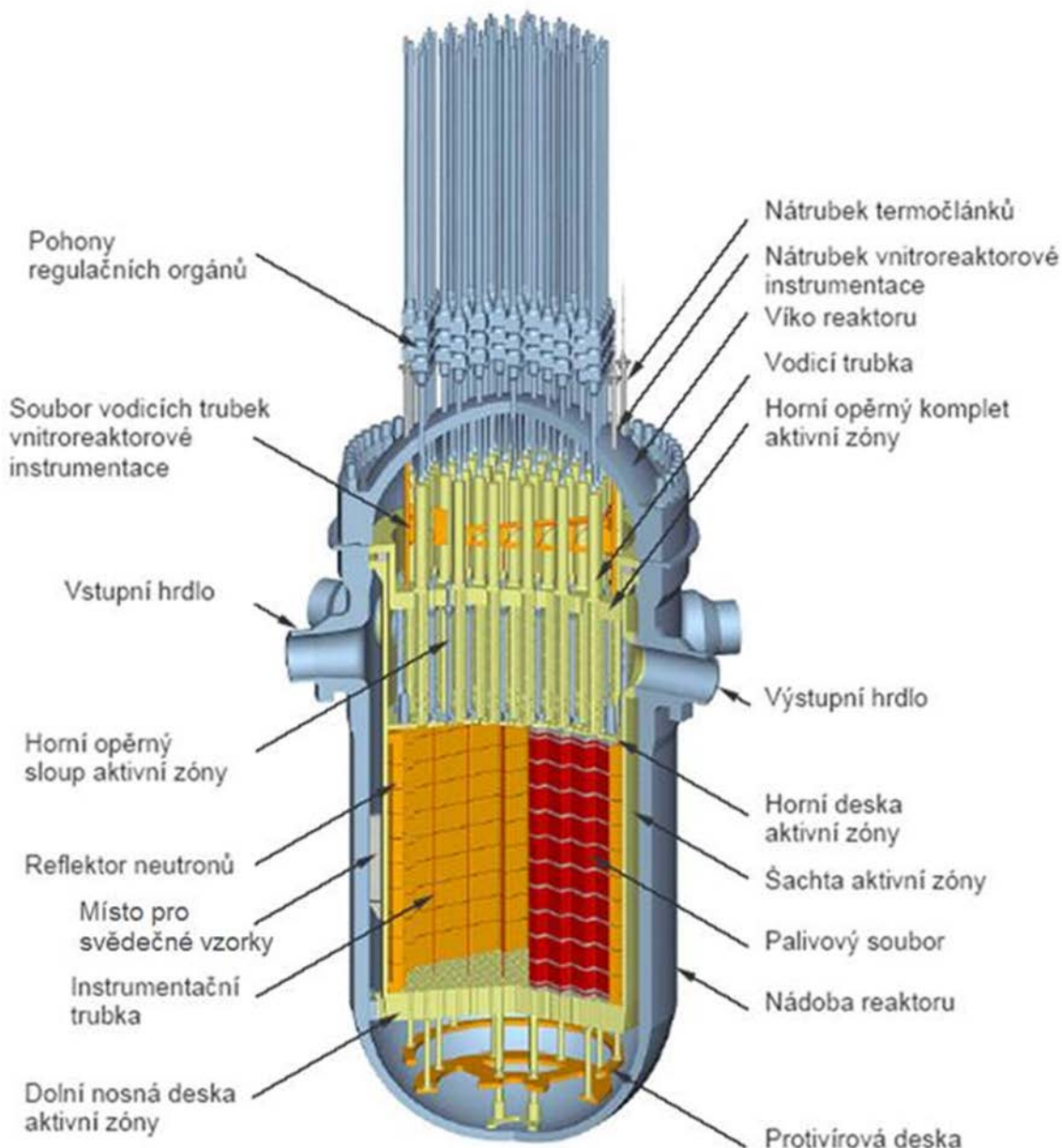
Obr. 49: Vertikální řez reaktoru VVER-1000
