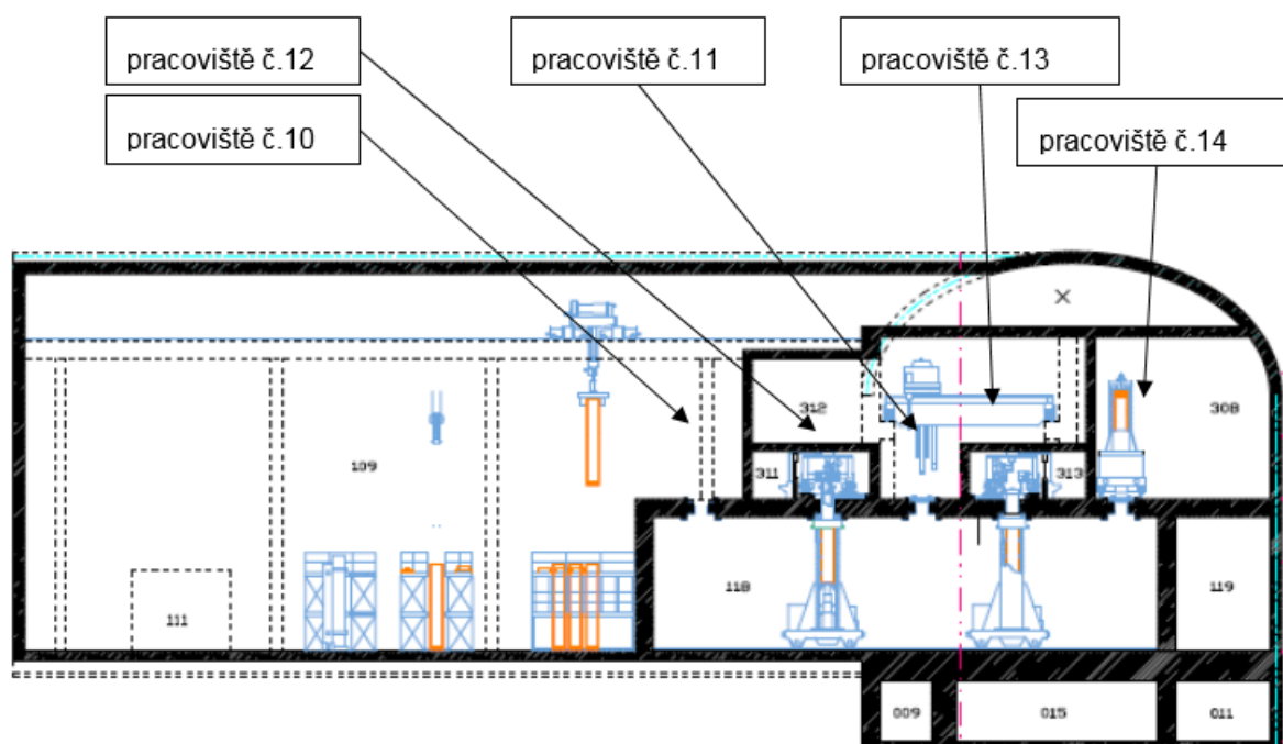
Obr. 69: Pracoviště zavážení VJP
