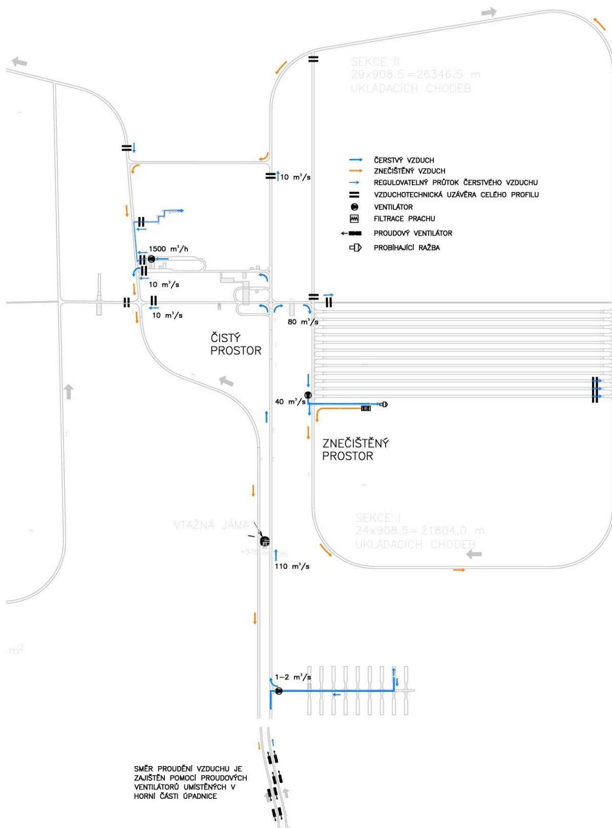
Obr. 63: Koncepční schéma větrání HÚ při ražbách pomocí TBM zavážecích chodeb a zavážení VJP do úložiště v sekci I.
