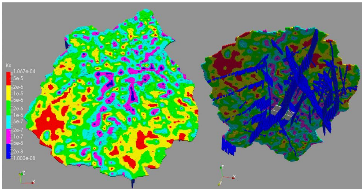
Obr. 15: Rozložení hodnot koeficientu hydraulické vodivosti vyšších než 1 \cdot 10^{-8} \text{ m.s}^{-1}
