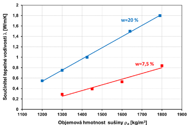
Obr. 55: Součinitel tepelné vodivosti pro bentonit B75 v závislosti na zhutnění
