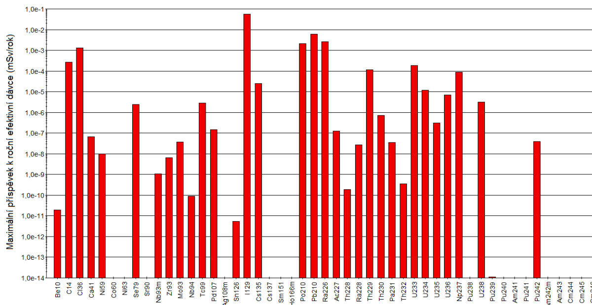
Maximální příspěvky radionuklidů k roční efektivní dávce (mSv/rok)
