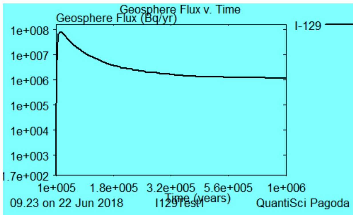
Obr. 45: Odhad toku I-129 do životního prostředí při okamžitém poškození všech obalových souborů
