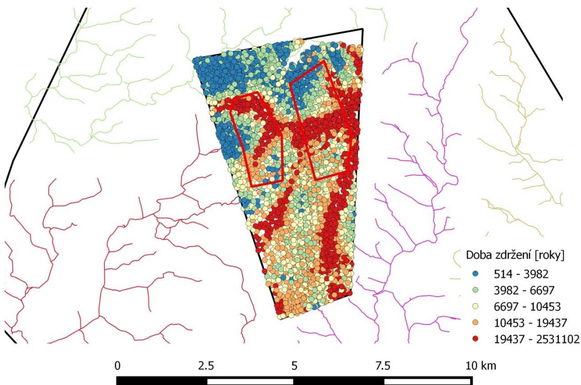
Obr. 21: Doby zdržení pro jednotlivé transportní cesty (Flow 123D)
