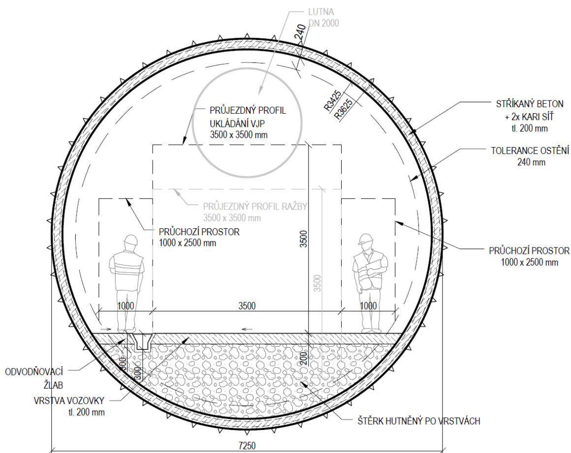
Obr. 66: Příčný řez zavážecím a odtěžovacím tunelem – pro variantu D1
