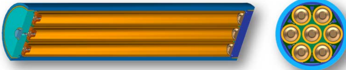
Obr. 51: Varianta UOS č. 12 (pro 7 PK VVER 440, vnější obal z uhlíkové oceli, sedm nerezových vnitřních pouzder a vestavba zajišťující vzájemnou polohu vnitřních pouzder)
