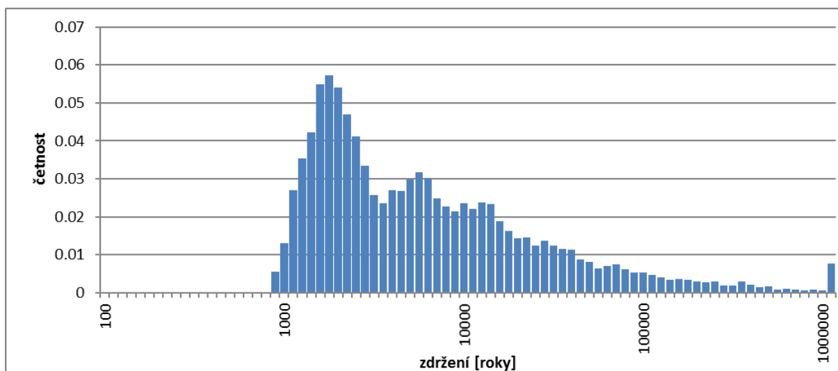
Obr. 19: Histogram doby zdržení částic v horninovém prostředí, homogenní blok západní, lokalita Čihadlo (MoldFlow)
