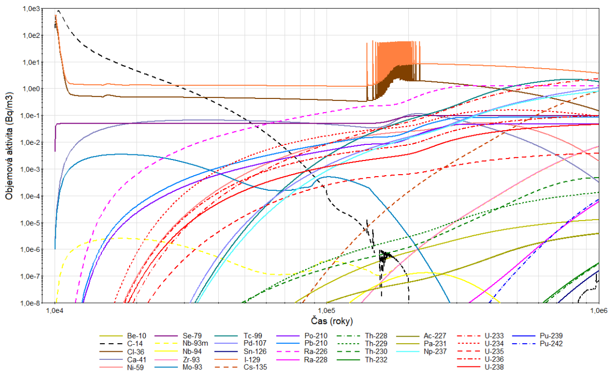
Obr. 41: Objemová aktivita radionuklidů v podzemní vodě na výstupu z geosféry (Bq/m 3 ) - (0-1000000 let)
