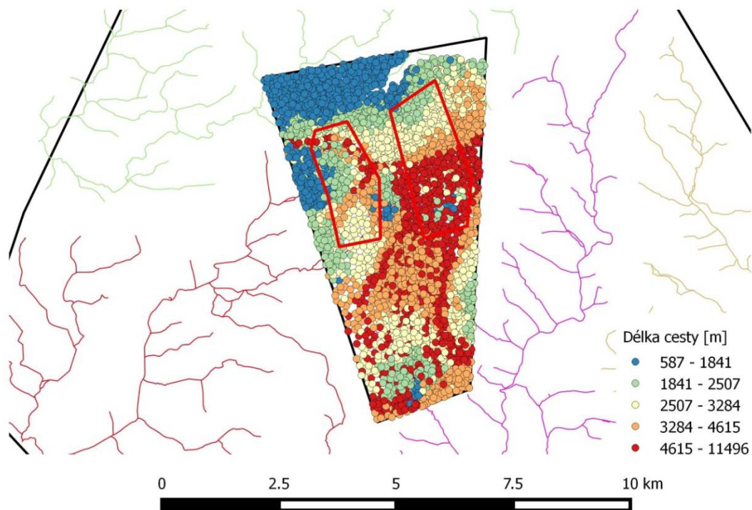
Obr. 20: Délky transportních cest v lokalitě Čihadlo (Flow 123D)
