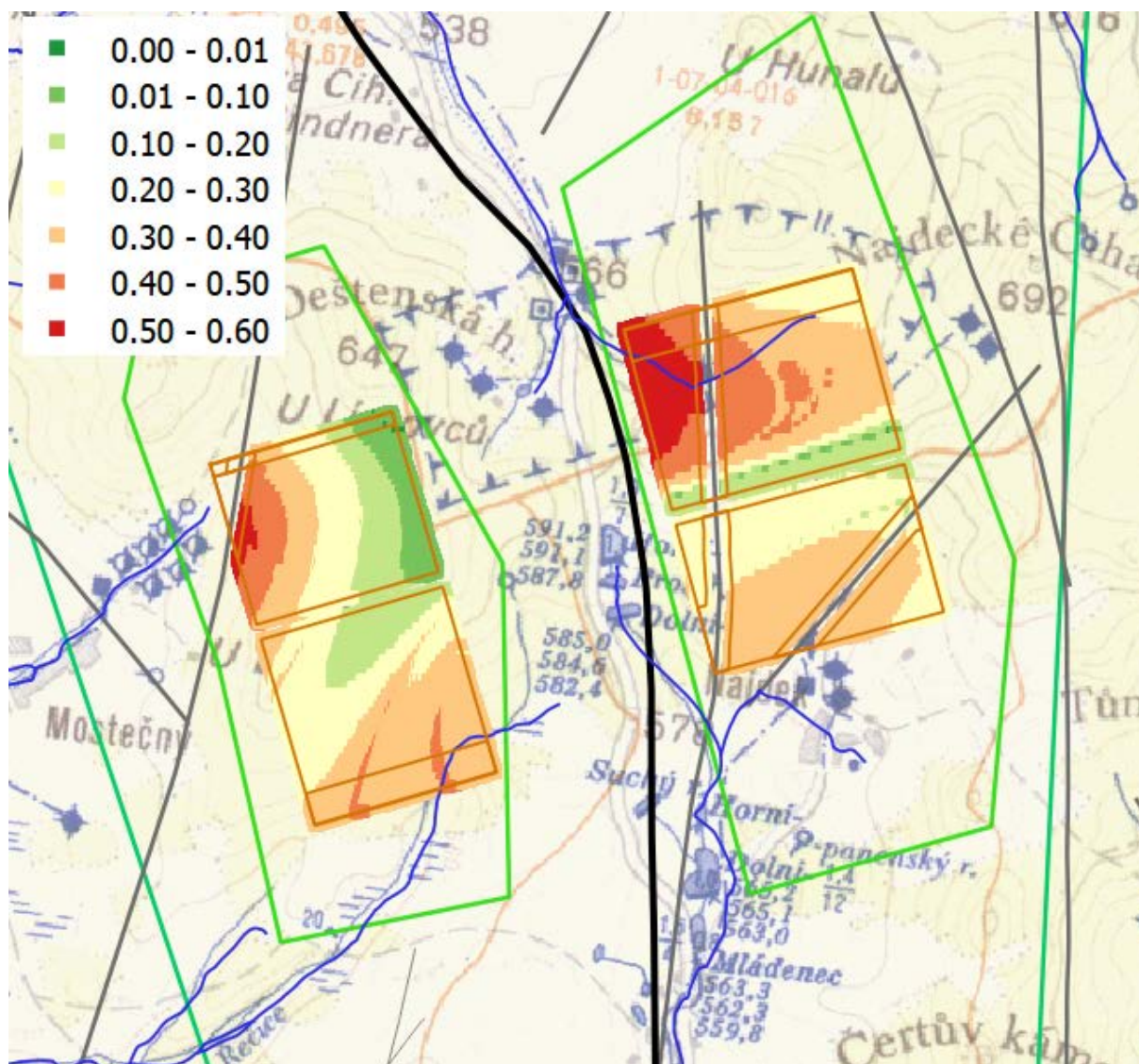
Obr. 16: Rozložení průměrných rychlostí proudění v [m.rok-1] z prostoru HÚ v modelu proudění
