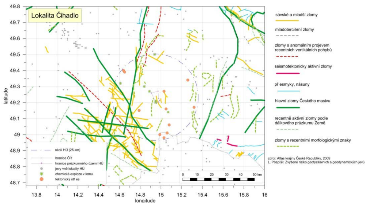
Obr. 22: Výřez z mapy „Zvýšené riziko geofyzikálních a geodynamických jevů“ (Hrnčiarová et al. 2009) s vyznačením potenciální lokality Čihadlo a okolí HÚ a seismickými jevy z databáze ČRSS
