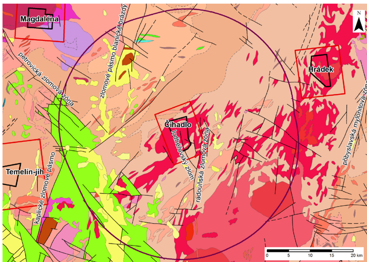
Obr. 6: Mapa zlomových struktur v širším okolí lokality Čihadlo (okruh 25 km od lokalizace zájmového území)
