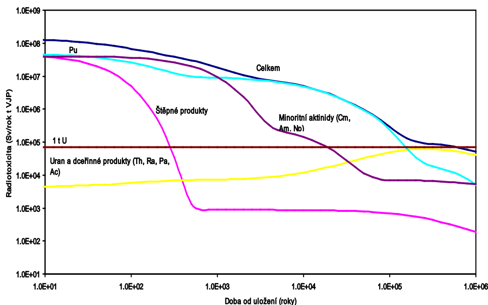
Obr. 31: Srovnání potencionální radiotoxicity vyhořelého jaderného paliva a jeho jednotlivých složek s potencionální radiotoxicitou 1 t uranové rudy.
