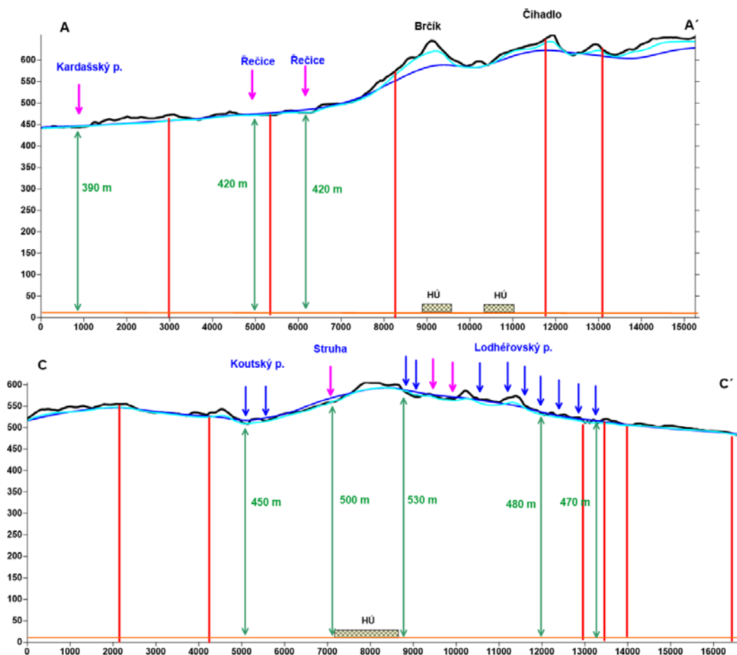
Obr. 13: Schématické řezy se znázorněním horizontální a vertikální vzdálenosti drenáže podzemní vody z prostoru projektovaného HÚ (fialové šipky) a homogenních bloků (modré šipky)
