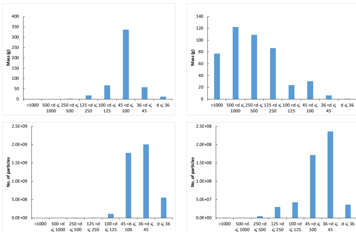
Obr. 1 Porovnání sítové analýzy vzorku bentonitu BCV (levá) a půdy z lokality Lítožnice (pravá): histogram hmotnostních frakcí (nahore) a po přepočtení na počty částic (dole)
